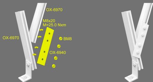
7. Instalación plato de fijación para cortavientos
