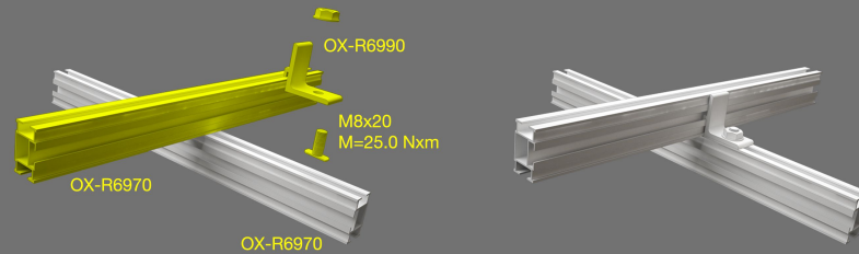
4. Montaje de Rail Omnia correa sobre Diagonal con Glimper
