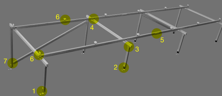
6. Montaje de Grounding Lug, Zeta y Omega clamp sobre Rail Omnia
