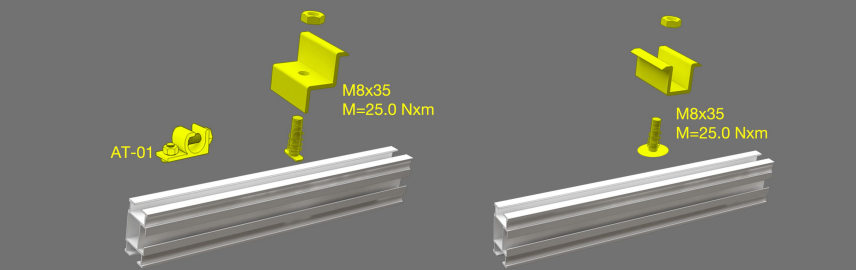
6. Montaje de Zeta y Omega clamp sobre Rail Omnia
