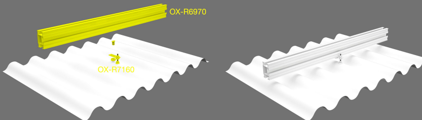
4. Detalle montaje de Rail Omnia sobre Tornillo
