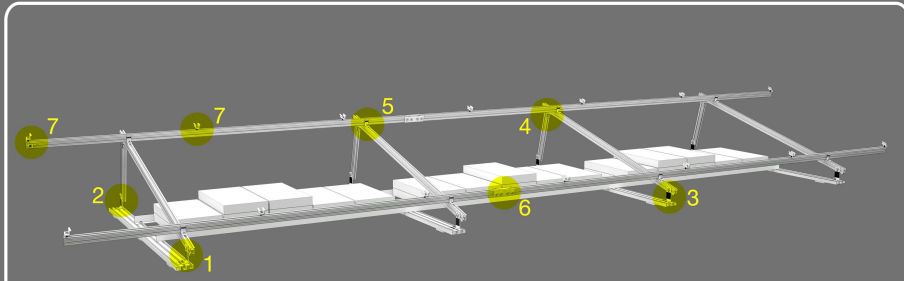
6. Montaje de Junction y Bonding jumper sobre Rail Omnia
