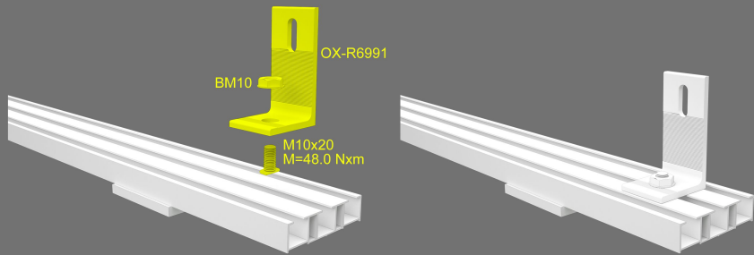
1. Montaje de L-FOOT sobre perfil Runner
