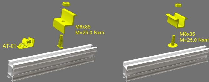
7. Montaje de Zeta y Omega clamp sobre Rail Omnia
