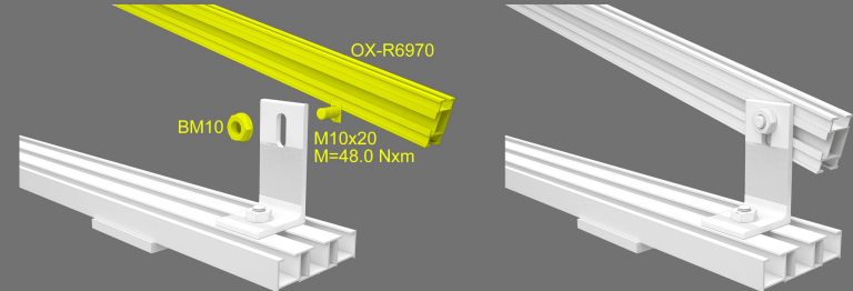
4. Montaje de Rail Omnia Diagonal sobre L-FOOT
