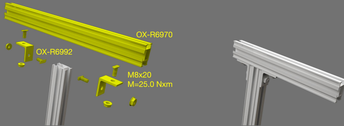
3. Montaje de Rail Omnia Diagonal con L-lock
