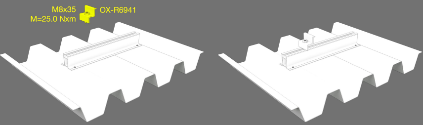
6. Montaje de Zeta clamp sobre MiniRail
