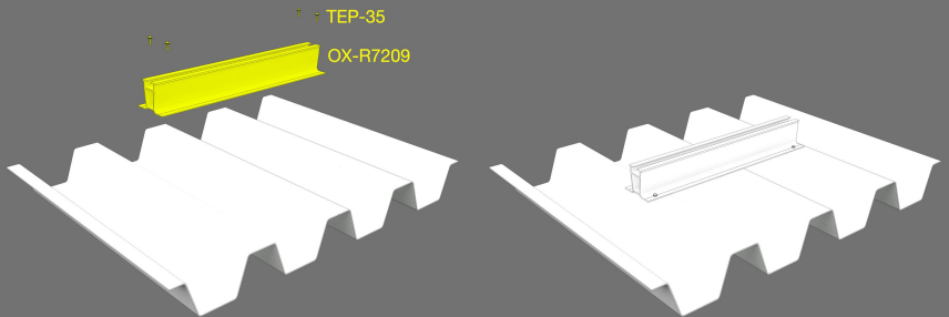
4. Fijación del MiniRail sobre lámina
