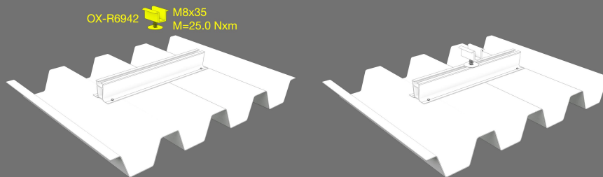
5. Montaje de Omega clamp sobre MiniRail
