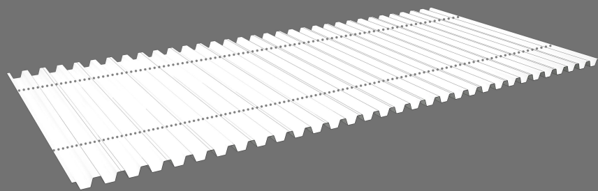
2. Marcar dos líneas de referencia para alinear todos los elementos estructurales
