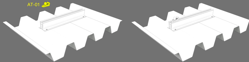
7. Montaje de Grounding sobre MiniRail
