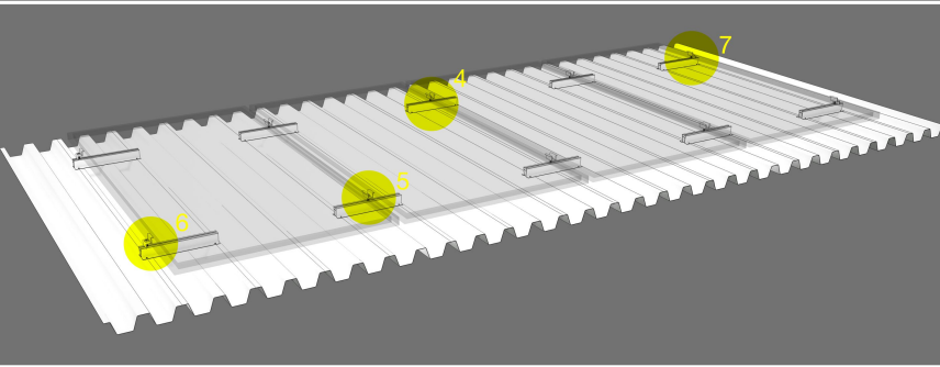
6. Montaje de Zeta clamp sobre MiniRail
