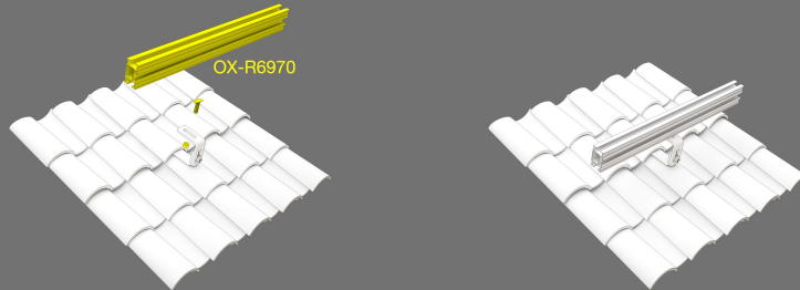
5. Detalle montaje de Rail Omnia sobre Roof Hook
