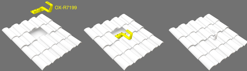
3. Detalle montaje de Roof Hook sobre techo
