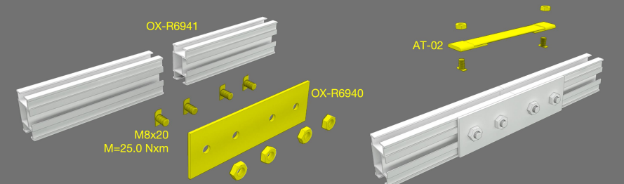
6. Montaje de Junction Omnia y Bonding jumper sobre Rail Omnia
