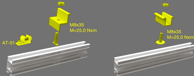
7. Montaje de Zeta, Omega clamp y Grounding sobre Rail Omnia
