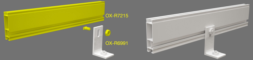
2. Montaje de Rail Ace sobre L-FOOT
