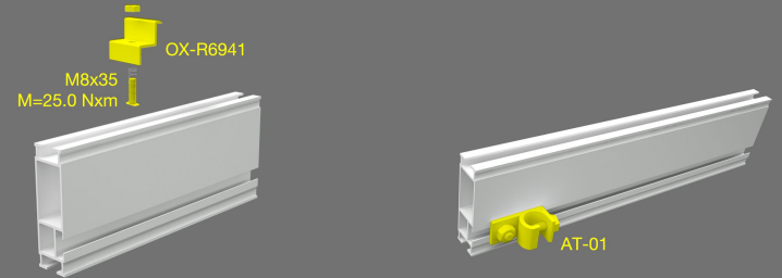
6. Instalación de Zeta Clamp y Grounding sobre Rail Ace
