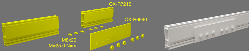
3. Montaje de Junction para Rail Ace
