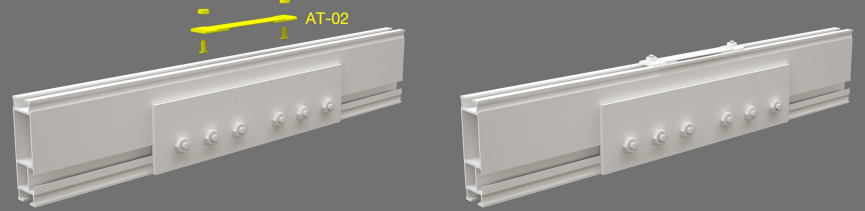
4. Montaje de Bonding Jumper sobre Rail Ace
