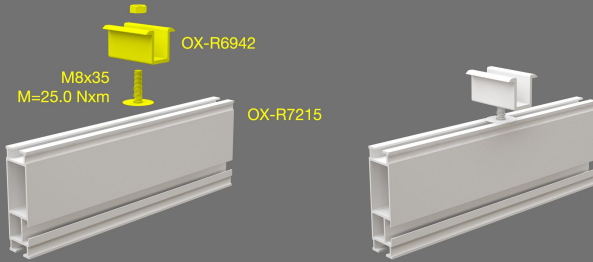
5. Instalación de Omega clamp sobre Rail Ace
